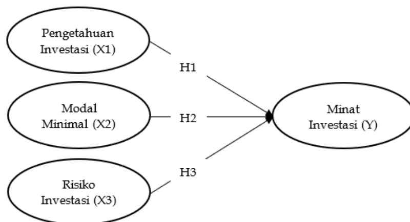
Gambar 1. Kerangka Penelitian
